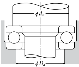
Fig. 11.3 Diámetro de los Apoyos para Rodamientos de Empuje de Bolas
