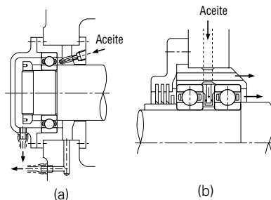
Fig. 12.8 Lubricación por Chorro
