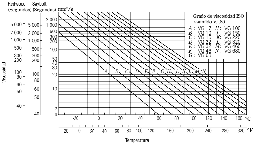
Fig. 12.11 Diagrama Temperatura-Viscosidad
