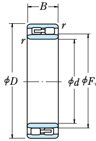
NNU Diámetro Interior Cilíndrico
