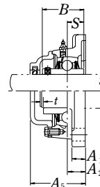
Tipo de cubierta de fundición anti polvo
