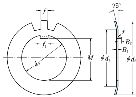
Aleta Doblada
