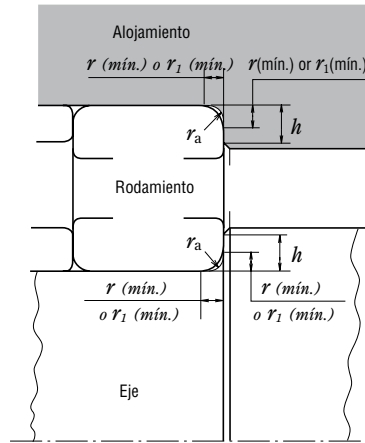
Fig. 11.1 Dimensiones del Chaflán del Rodamiento, Radio del Chaflán de Eje y Alojamiento, y Altura del Codo
