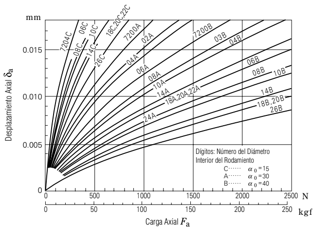
Fig. 15.3 Carga Axial y Desplazamiento Axial de Rodamientos de Bolas de Contacto Angular
