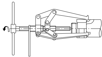
Fig. 14.14 Extracción del Anillo Interior Utilizando una Herramienta de Desmontaje (2)
